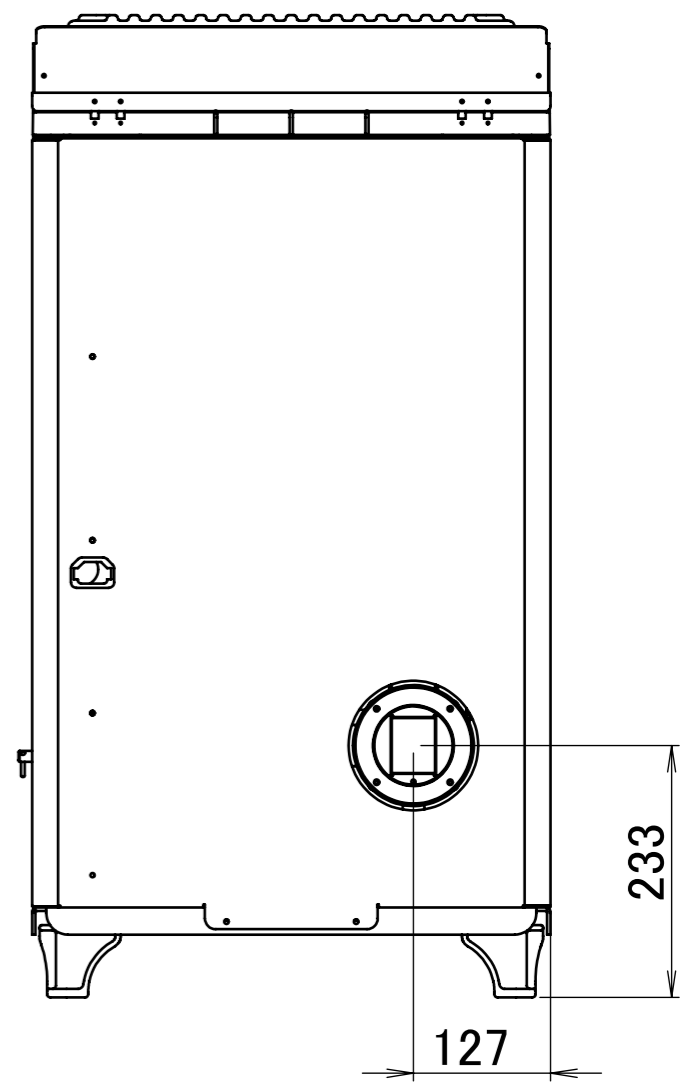
SAIKAI RS-4 外觀寸法図
